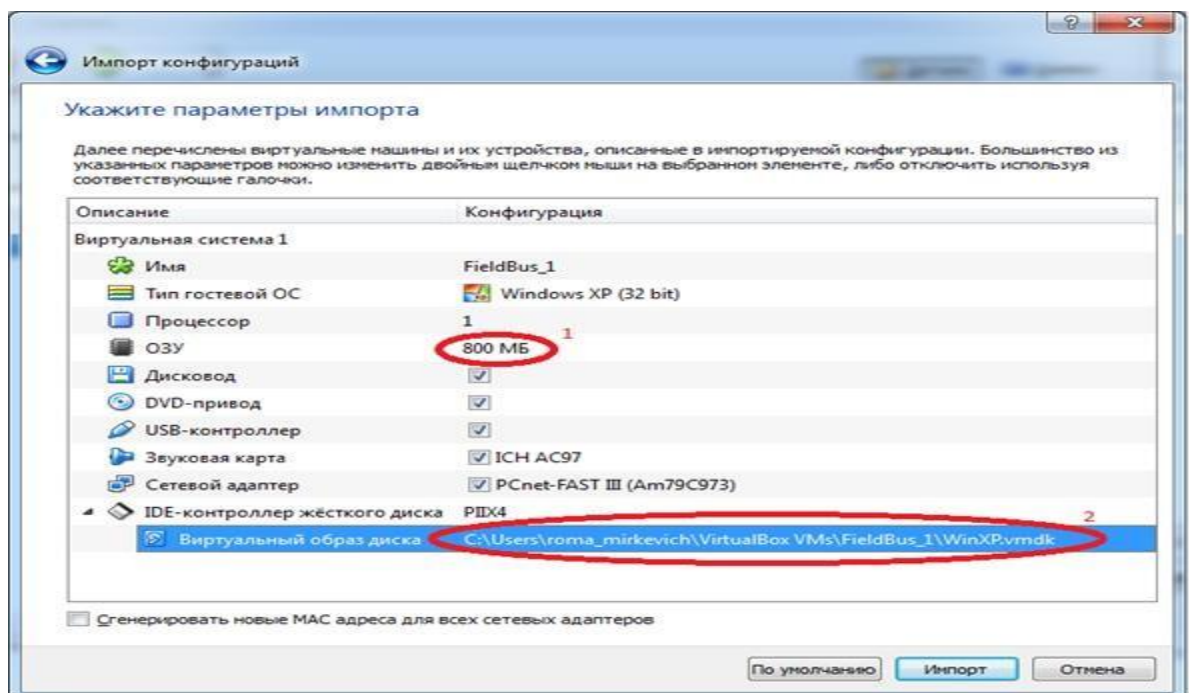
Рис.6. Налаштування параметрів конфігурації
